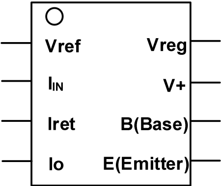
图-A 管脚定义 (Top view)
